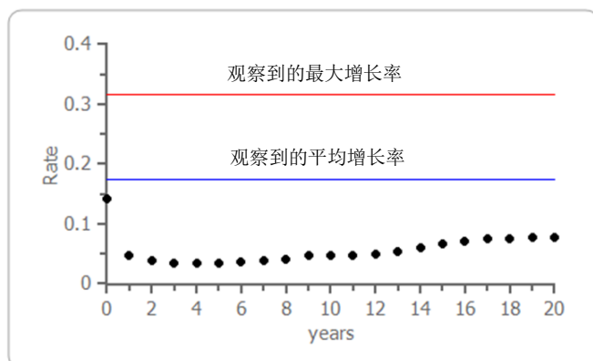
目标规模=500
