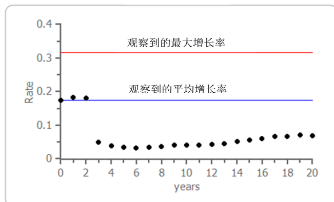
目标规模=600
